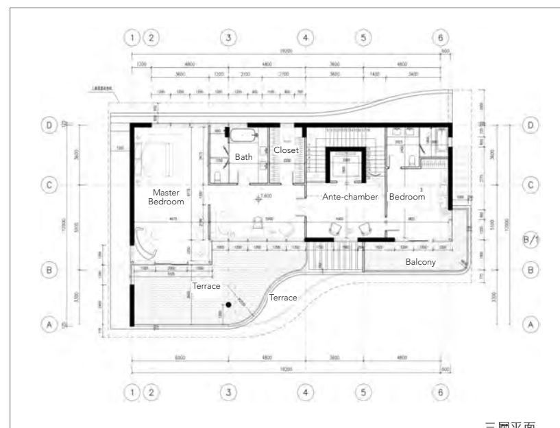
三層平面
