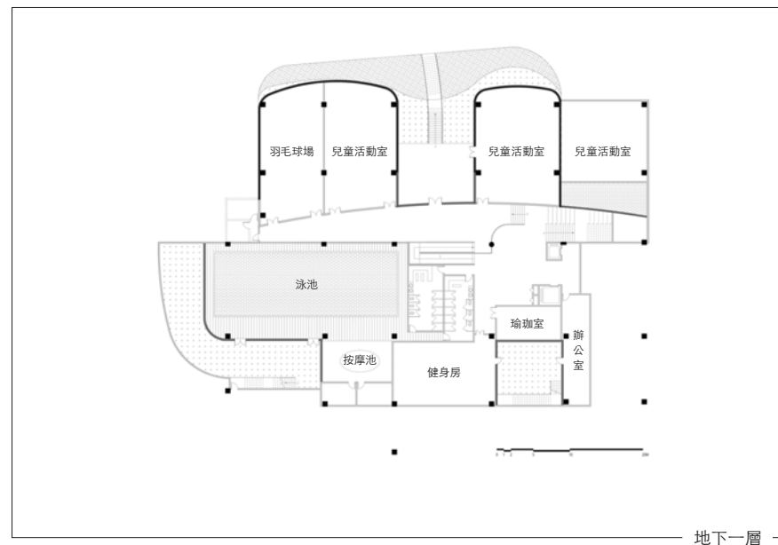
地下一層
