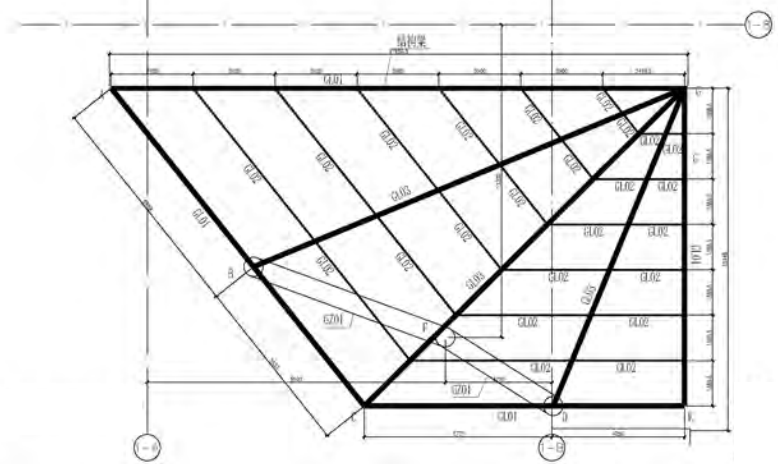
W 雨蓬構造圖
