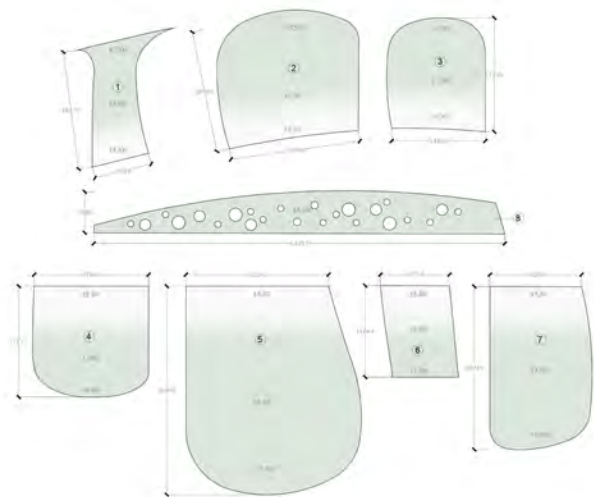
屋頂放樣圖
