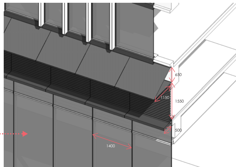
雨蓬及簷口大樣
