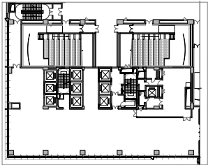
五層
