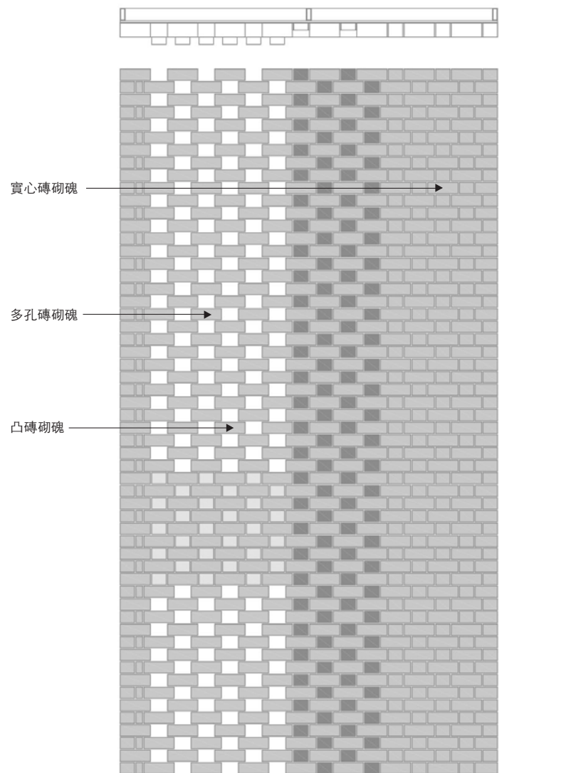
黏土磚掛幕詳圖
