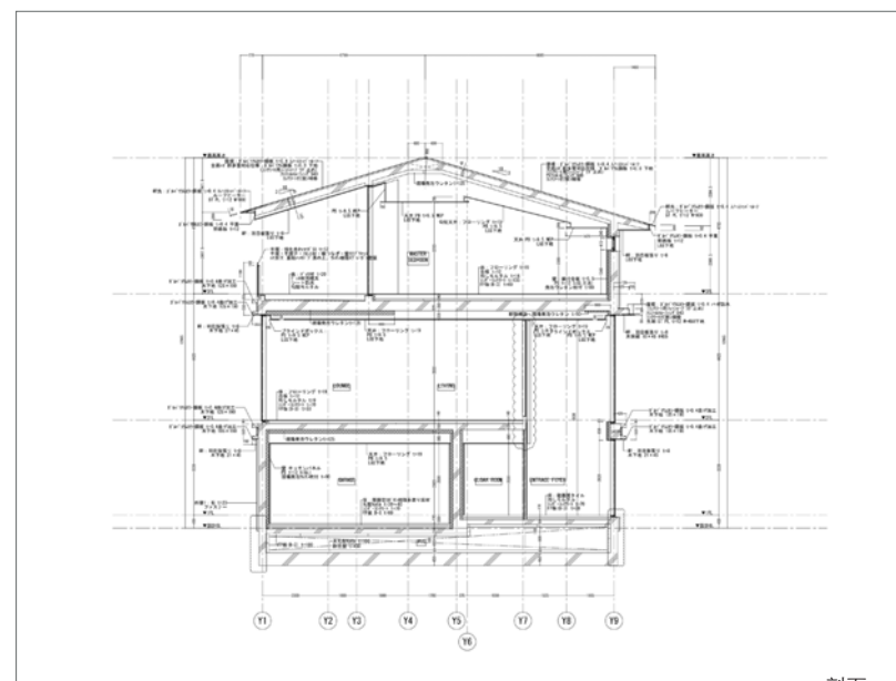
剖面
