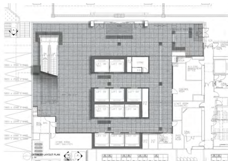
▲ 大堂平面
