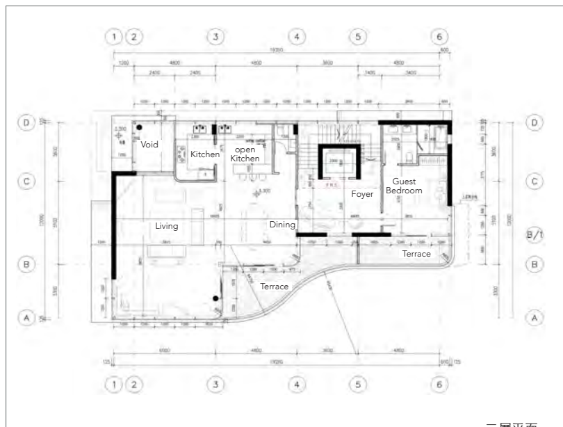
二層平面
